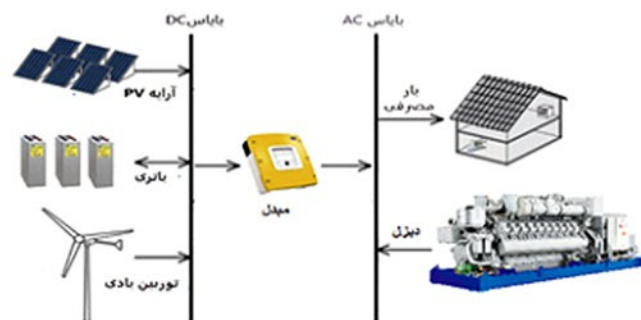
شکل ۱. شماتیک سیستم هیبریدی
