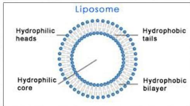
شکل ۱- ساختار لیپوزوم
