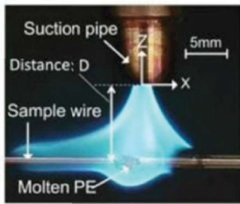
شکل ۵ - اطفاء حریق با مکش [۱۰]
